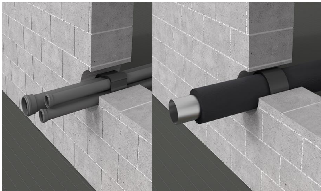
Rysunek 4.4: Możliwe zastosowania taśm ogniochronnych INTU FR WRAP L
