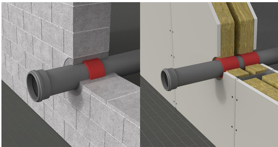
Rysunek 4.2: Możliwe zastosowania opasek ogniochronnych INTU FR WRAP
